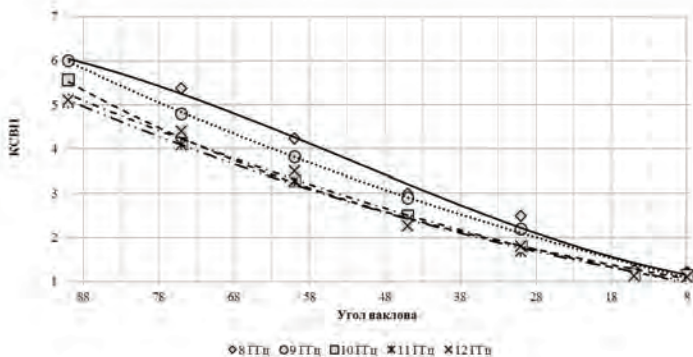
Рисунок 2 - Зависимость КСВН от угла наклона стенки измерительной кюветы.
