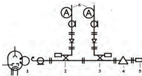
1 - ЛОВ; 2, 3– волноводные направленные ответвители падающей и отраженной волны; 4 - измерительная ячейка; 5 – согласованная
